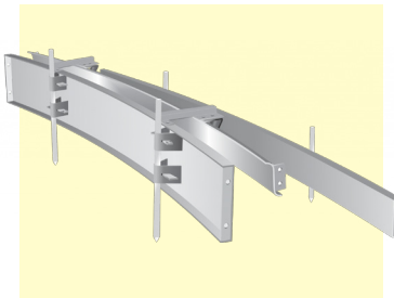
Bocacalle Cordón Cuneta Curvo Respaldo Enterizo
