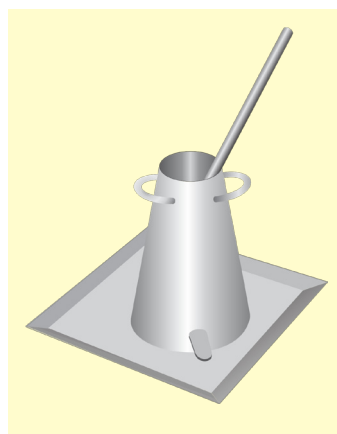
Cono de Abrams
