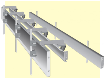
Cordón Cuneta Recto Respaldo Enterizo
